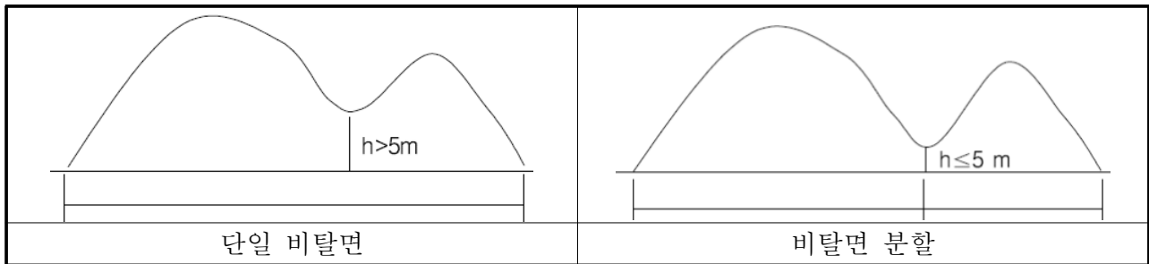
<그림 2.2-1> 절토비탈면 분할 기준
