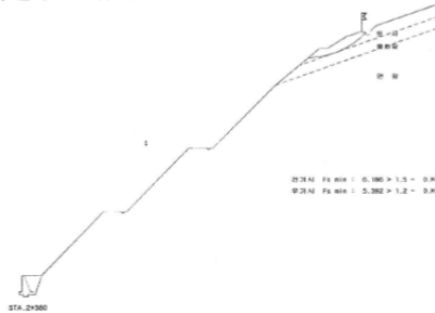
&lt;그림 4.21&gt; 범물지구~고산국도간 도로 STA.2+380 좌측 토사사면 안정검토
