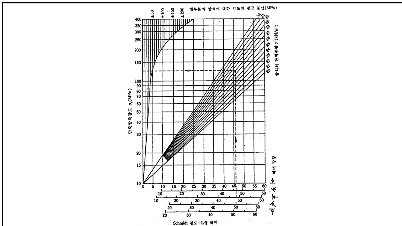
〈그림 2.2-2〉 슈미트해머 반발지수를 이용한 일축압축강도 변환 차트
