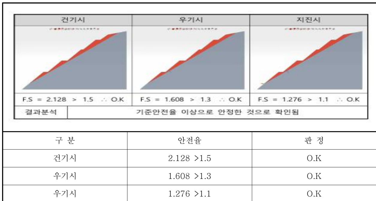
〈그림 2.4-5〉 한계평형해석
